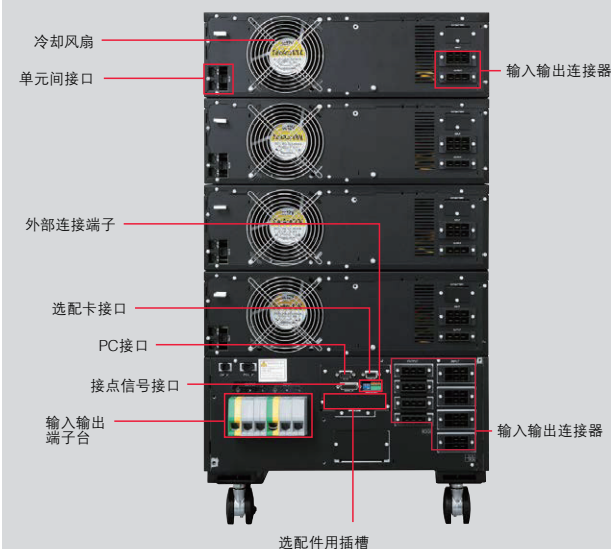
20kVA UL·CE认证产品 背面 型号名称：A11J203S****U
