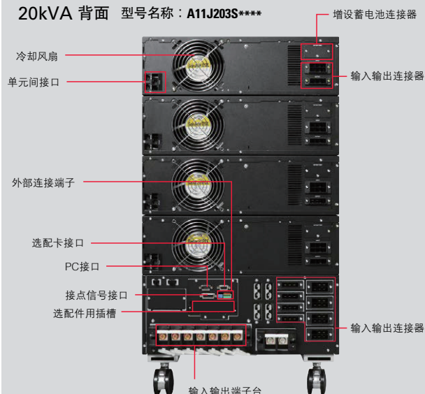
20kVA 背面 型号名称：A11J203S****
