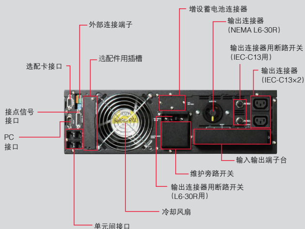
5kVA 背面 型号名称：A11J502****T 端子台型
